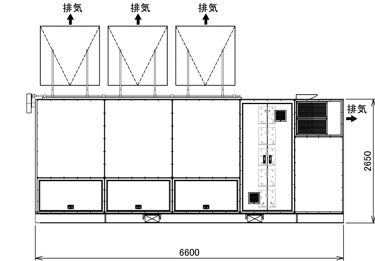
左側面図
