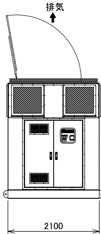
正面図
