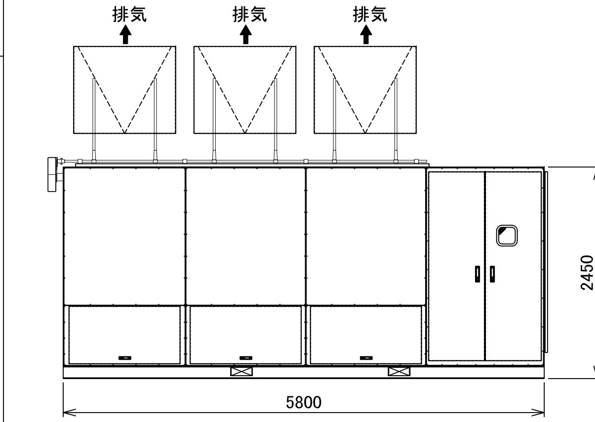
左側面図
