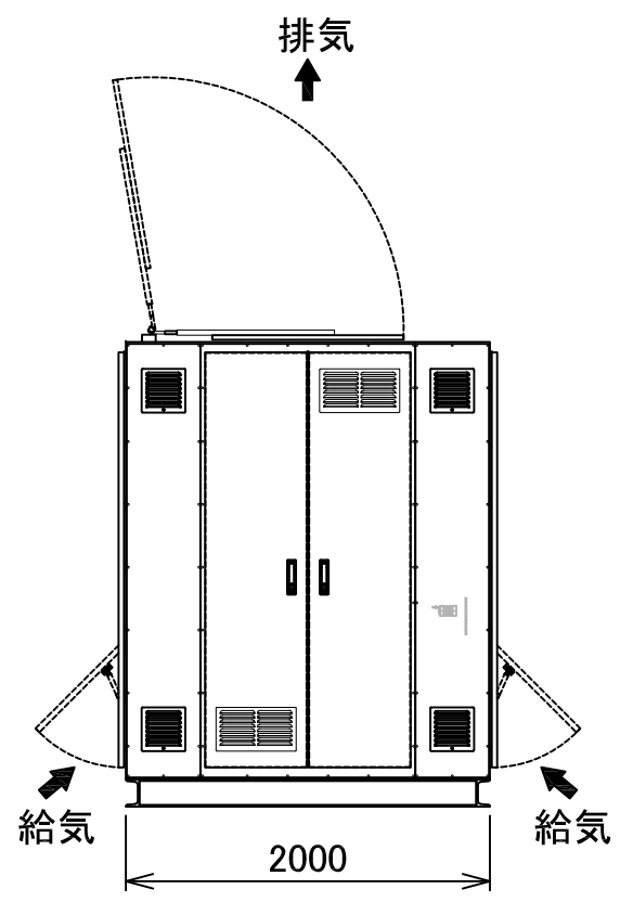
正面図
