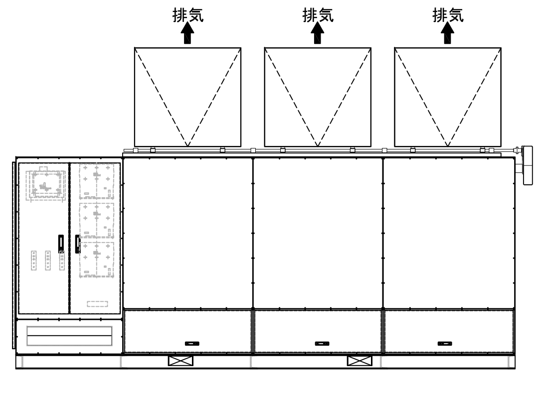
右側面図
