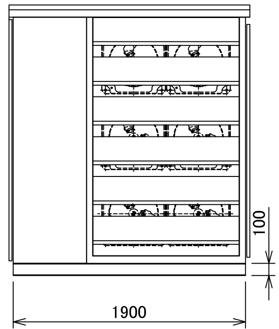
右側面図
