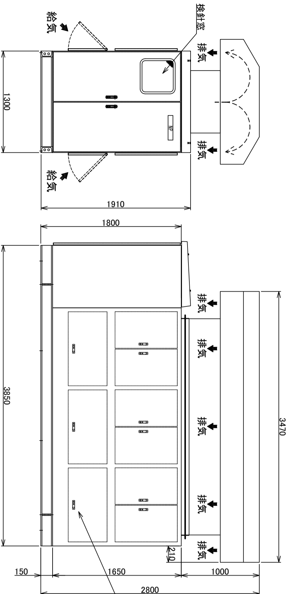
正面図
