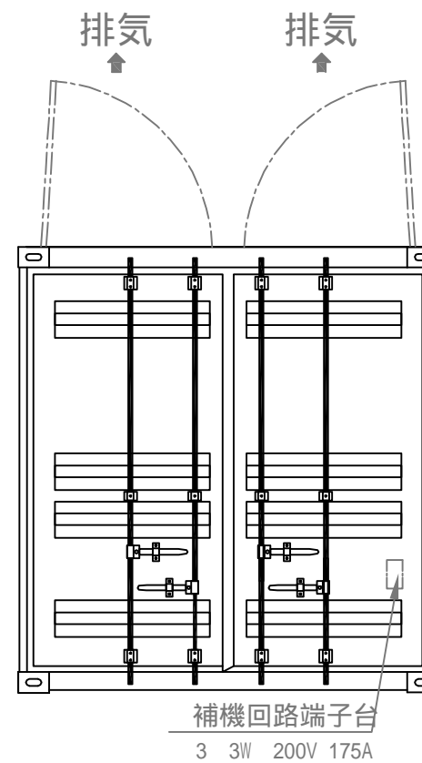
正面図
