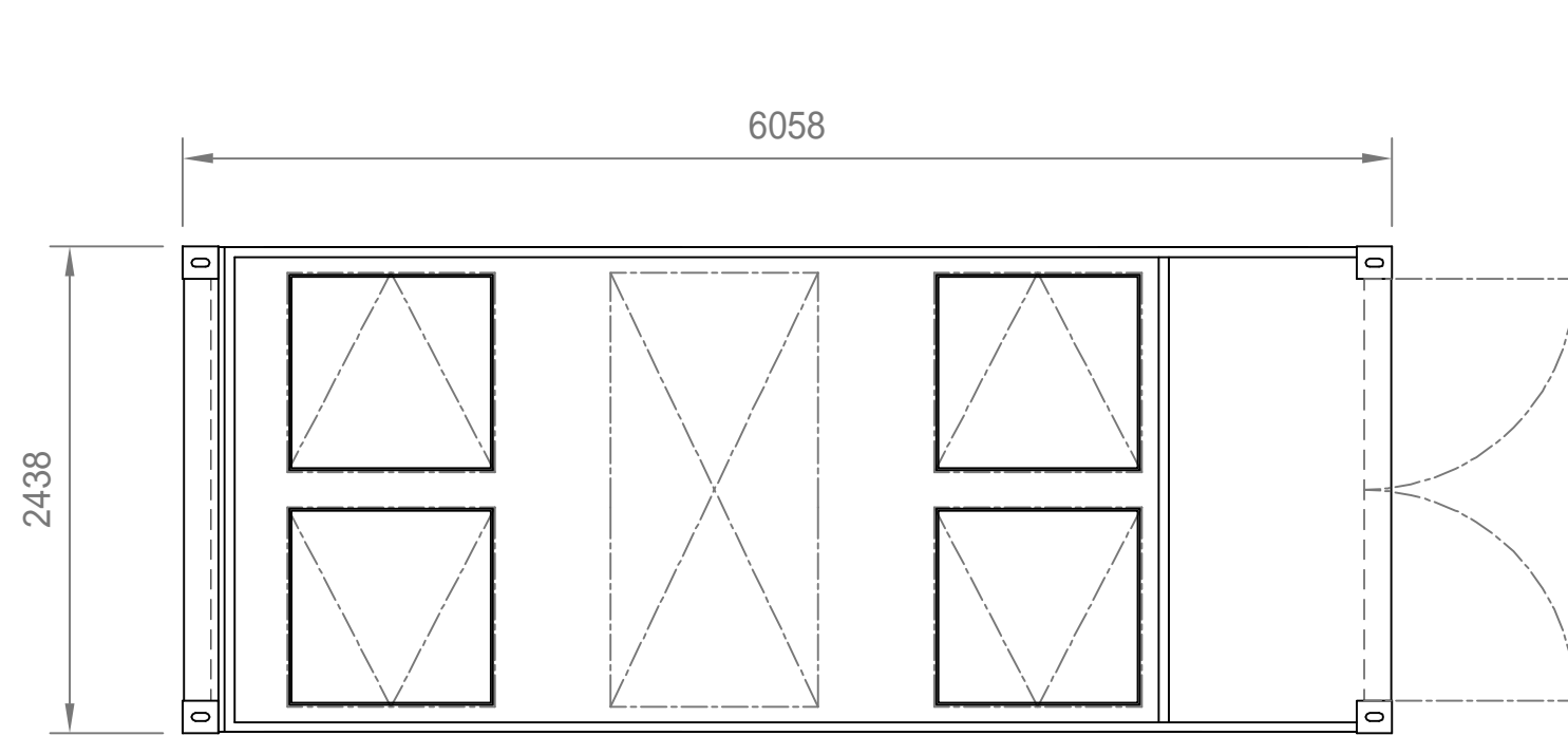
上面図
