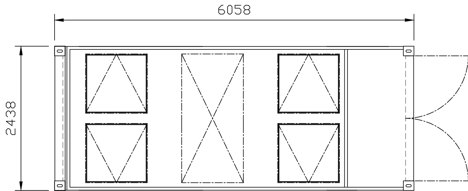
上面図
