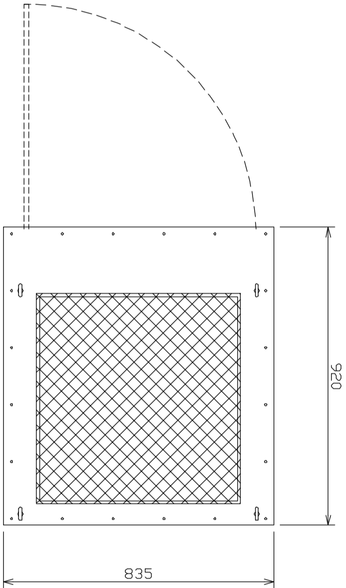
上面図
